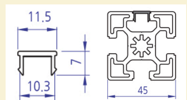
P/N: ES-CGR M8
