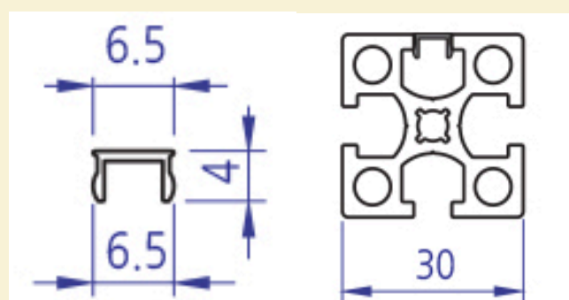
P/N: ES-CGR M6
